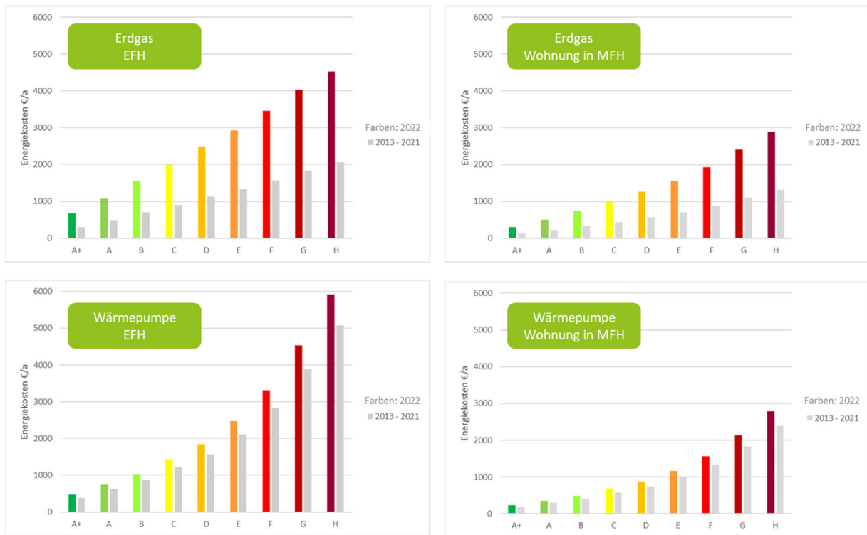
Abbildung 9: Heizkosten nach Effizienzklasse in 2022 und vor Ausbruch des Ukraine-Kriegs für Gasheizungen und Wärmepumpen für ein Einfamilienhaus und eine Wohnung (Annahme Wärmepumpen: Haushaltstarif)
